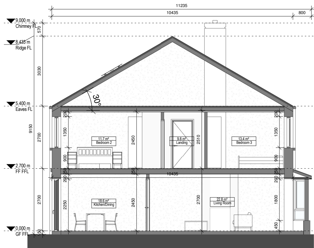
1 Section 1 1:100 @ A3
